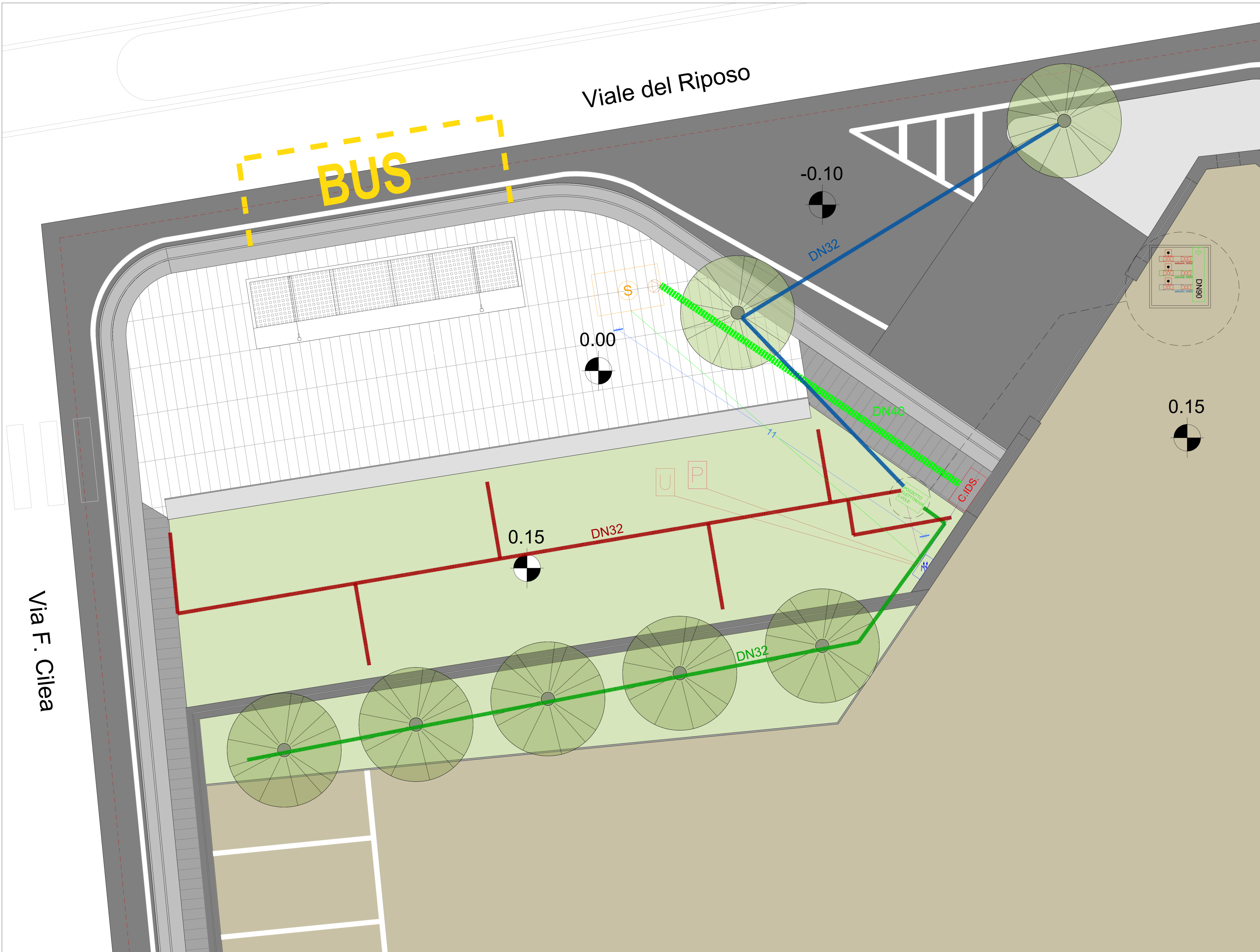
Stralcio planimetrico - scala 1:50
